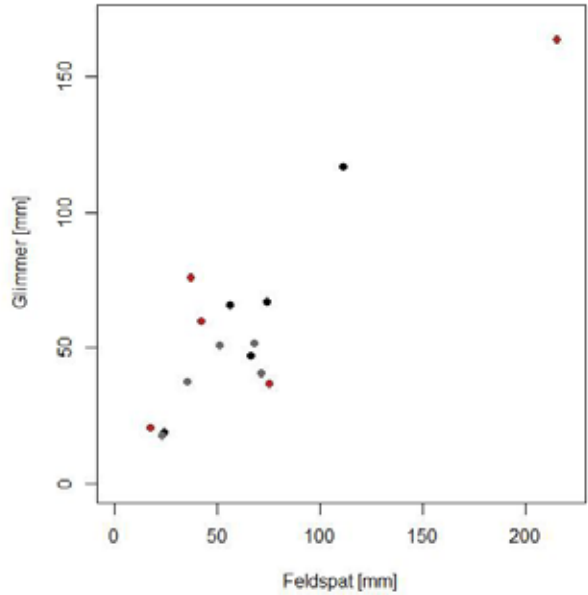
Diagramm 2: Intensitäten der Hauptpeaks von Glimmer zur Feldspatgruppe in mm (braun = bA-E, grau = gA-E, schwarz = sA-E)
